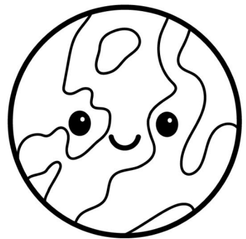
VENUS
