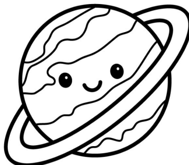
URANUS
