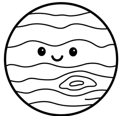
JUPITER
